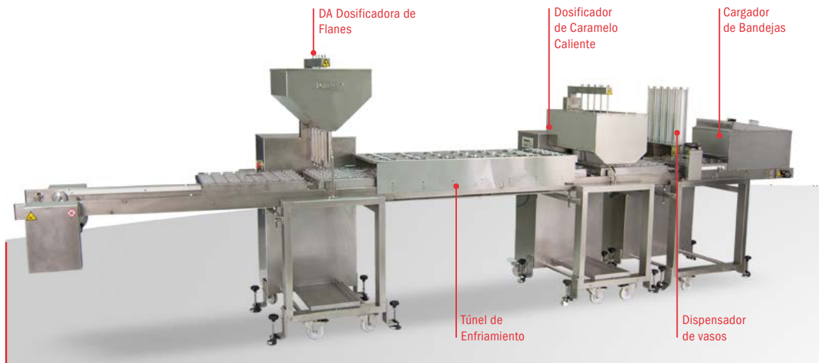
Línea Modular para la producción de flanes
