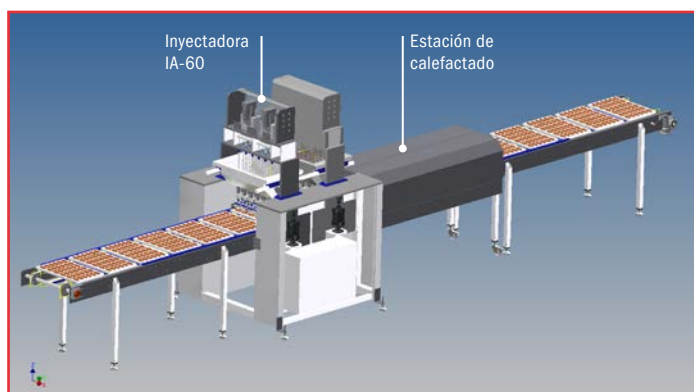
Línea modular para la inyección de croissants con doble depósito
